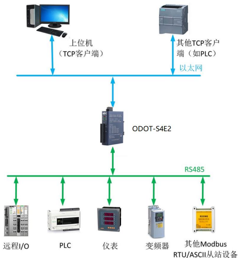
图 3.1 系统拓扑图
